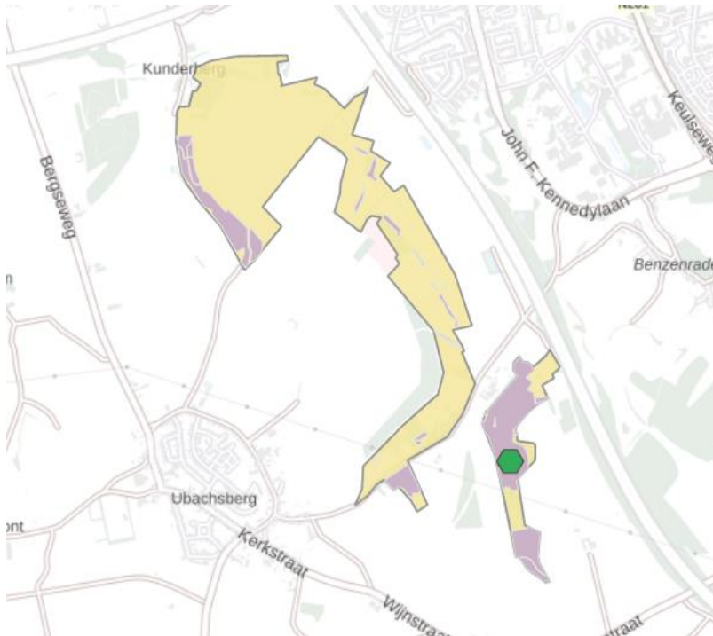
Kalktufbronnen 2020
