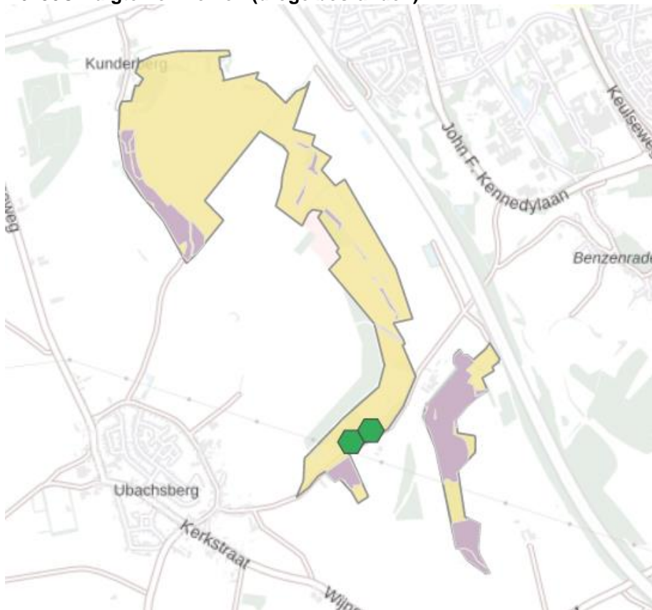
Kalkgrasland 2030
